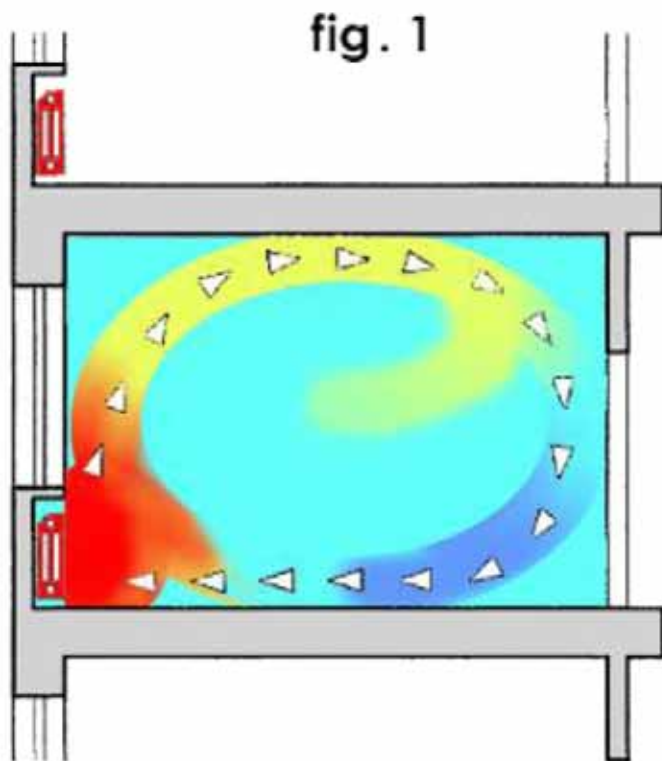
Moti convettivi in un impianto a radiatori
